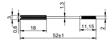
M2*2*52mm
